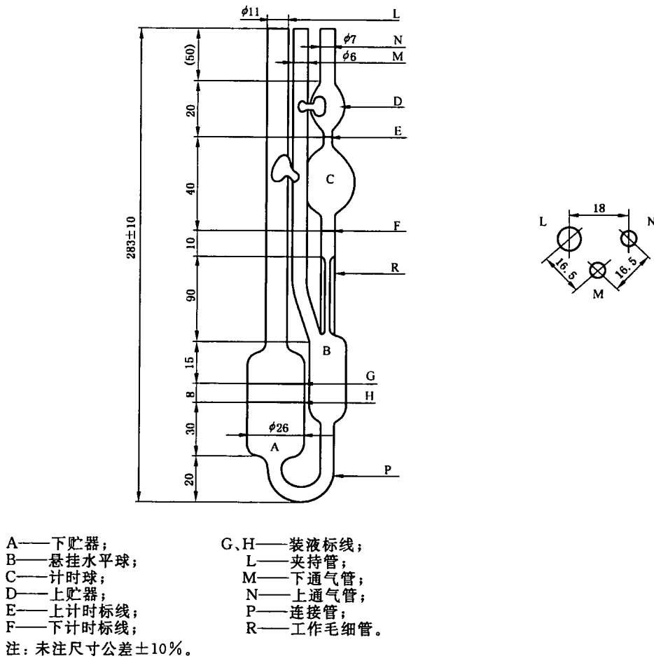
图 A.3 乌氏粘度计示意图
